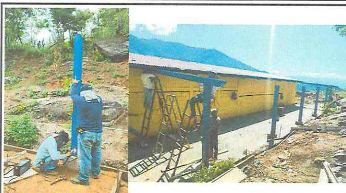
FOTO 2: INICIARON CON LA INSTALACIÓN DE LAS COLUMNAS Y VIGAS DE METAL CON COSTANERA DE METAL
